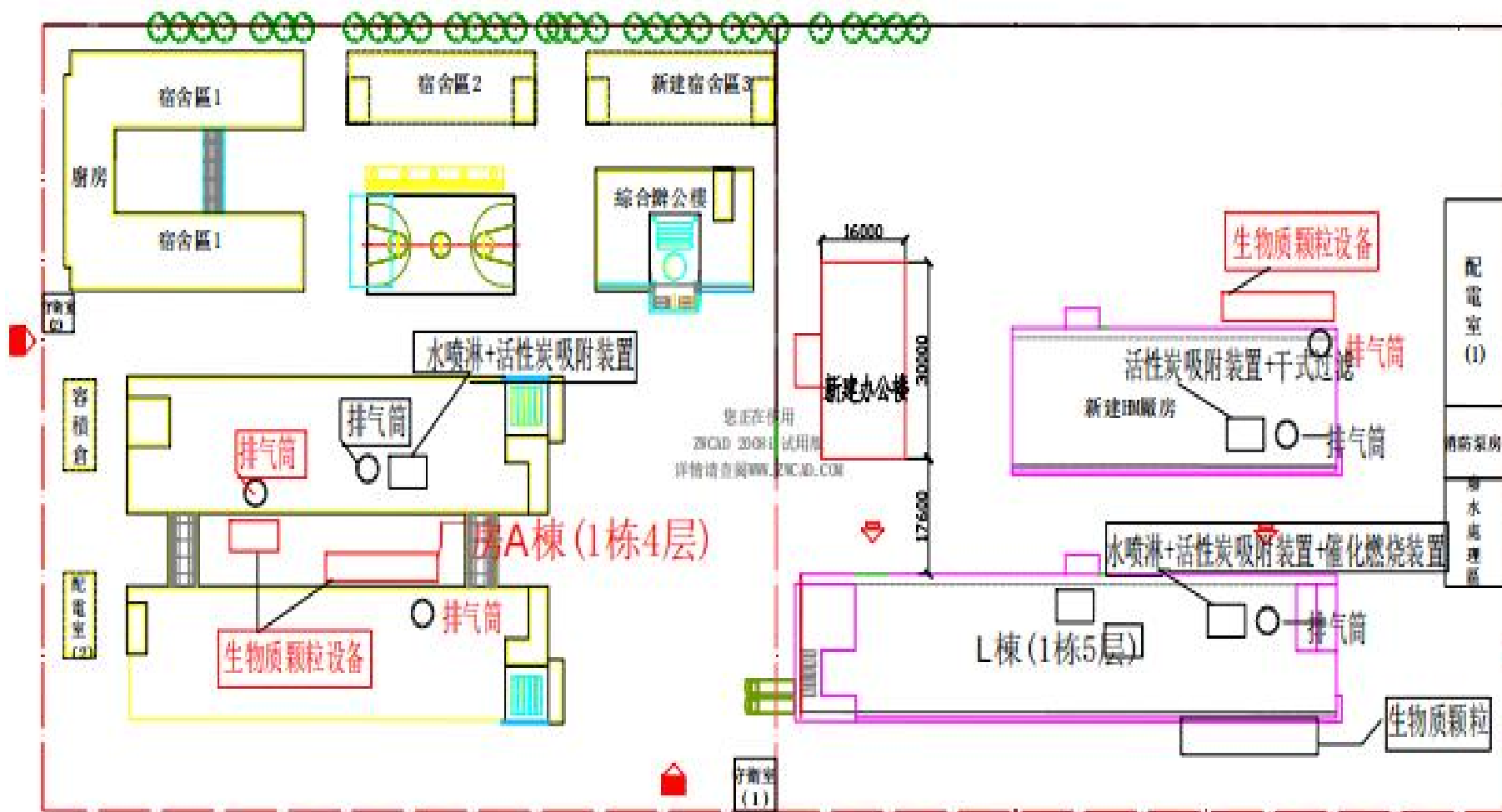
图 3-3 项目厂区总平面布局图
