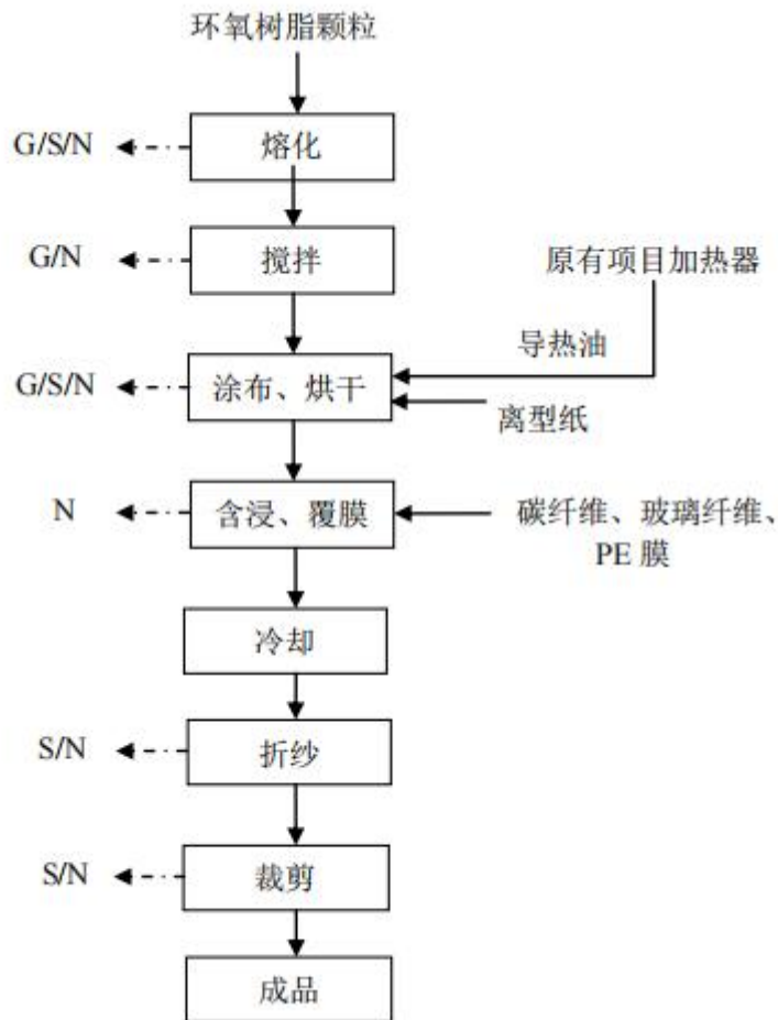
图1 织板工艺及产污环节流程示意图
